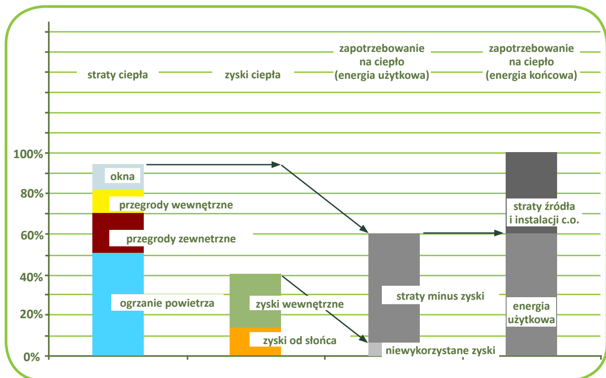
Rys. 14. Ilustracja strat i zysków ciepła oraz zapotrzebowania na energię użytkową i końcową Źródło: Fundacja Poszanowania Energii.
