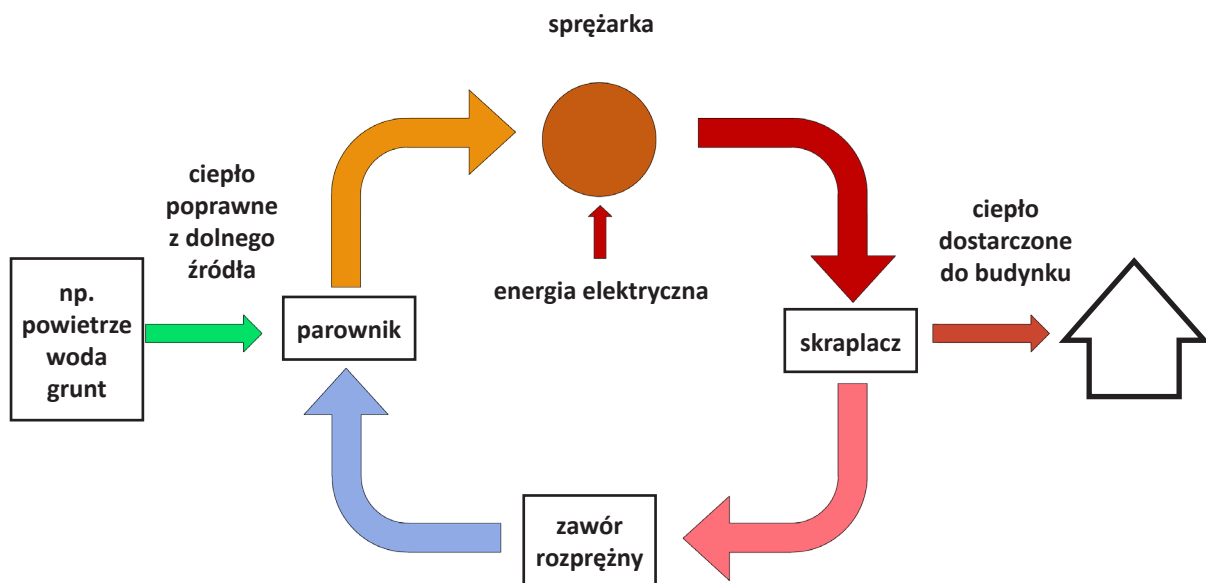
Rys. 38. Schemat działania pompy ciepła Źródło: Fundacja poszanowania Energii.
