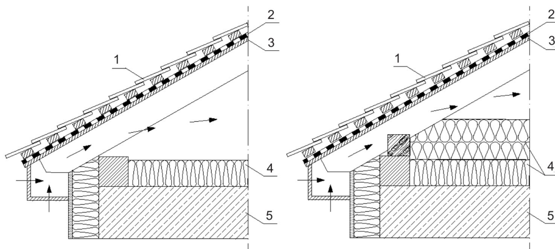
Rys. 24. Modernizacja dachu nad poddaszem nieużytkowym: 1 – pokrycie dachowe (dachówki), 2 – izolacja wodna i wiatroizolacja, 3 – podbitka, 4 – izolacja cieplna, 5 – strop Źródło: Fundacja Poszanowania Energii.
