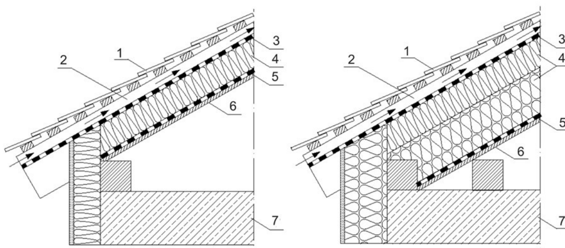
Rys. 25. Modernizacja dachu nad poddaszem użytkowym: 1 – pokrycie dachowe (dachówki), 2 – szczelina wentylacyjna (2-3 cm grubości), 3 – folia paroprzepuszczalna, 4 – izolacja cieplna, 5 – membrana paroszczelna (tylko w pomieszczeniach „mokrych”), 6 – wykończenie (np. drewno), 7 – strop Źródło: Fundacja Poszanowania Energii.
