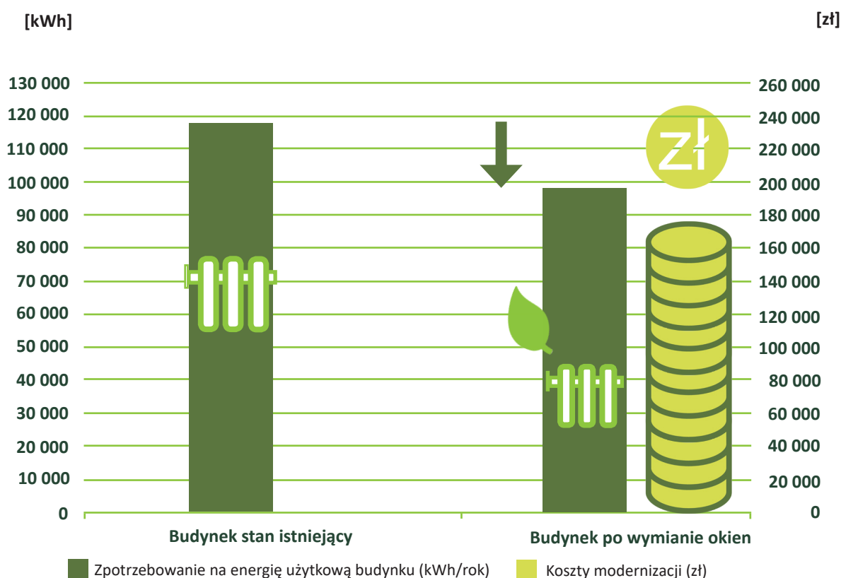
Rys. 29. Przykładowy wpływ modernizacji okien na zapotrzebowanie na energię użytkową do ogrzewania i koszty modernizacji (więcej informacji o założeniach do obliczeń w załączniku nr 1) Źródło: Fundacja Poszanowania Energii.
